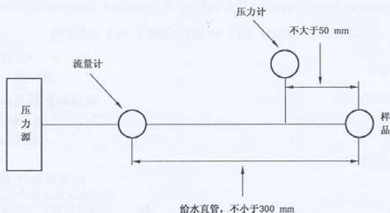
图 1 冲洗性能试验装置
