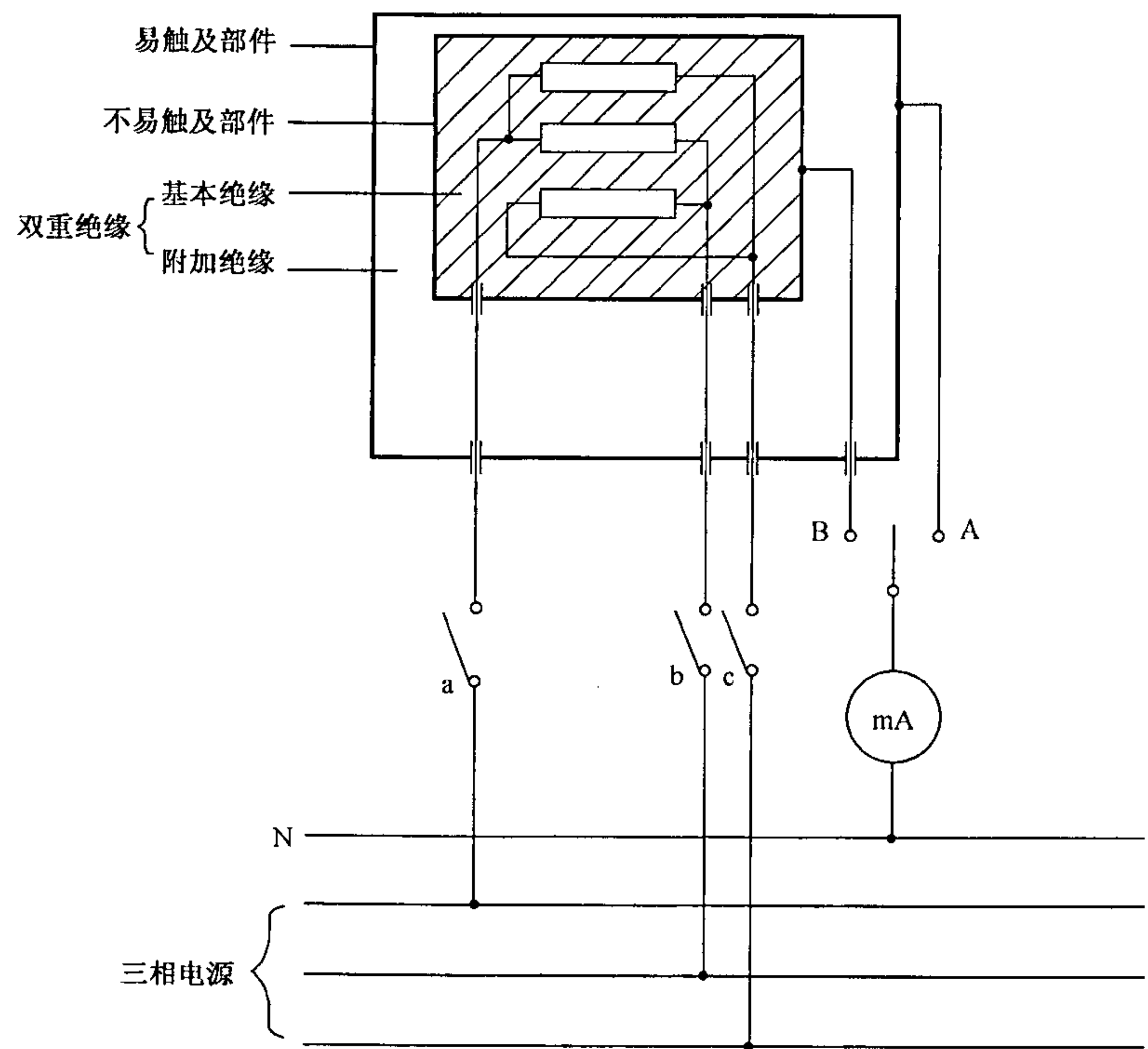
图 27 在工作温度下测量Ⅱ类控制器在三相连接时泄漏电流的接线图
