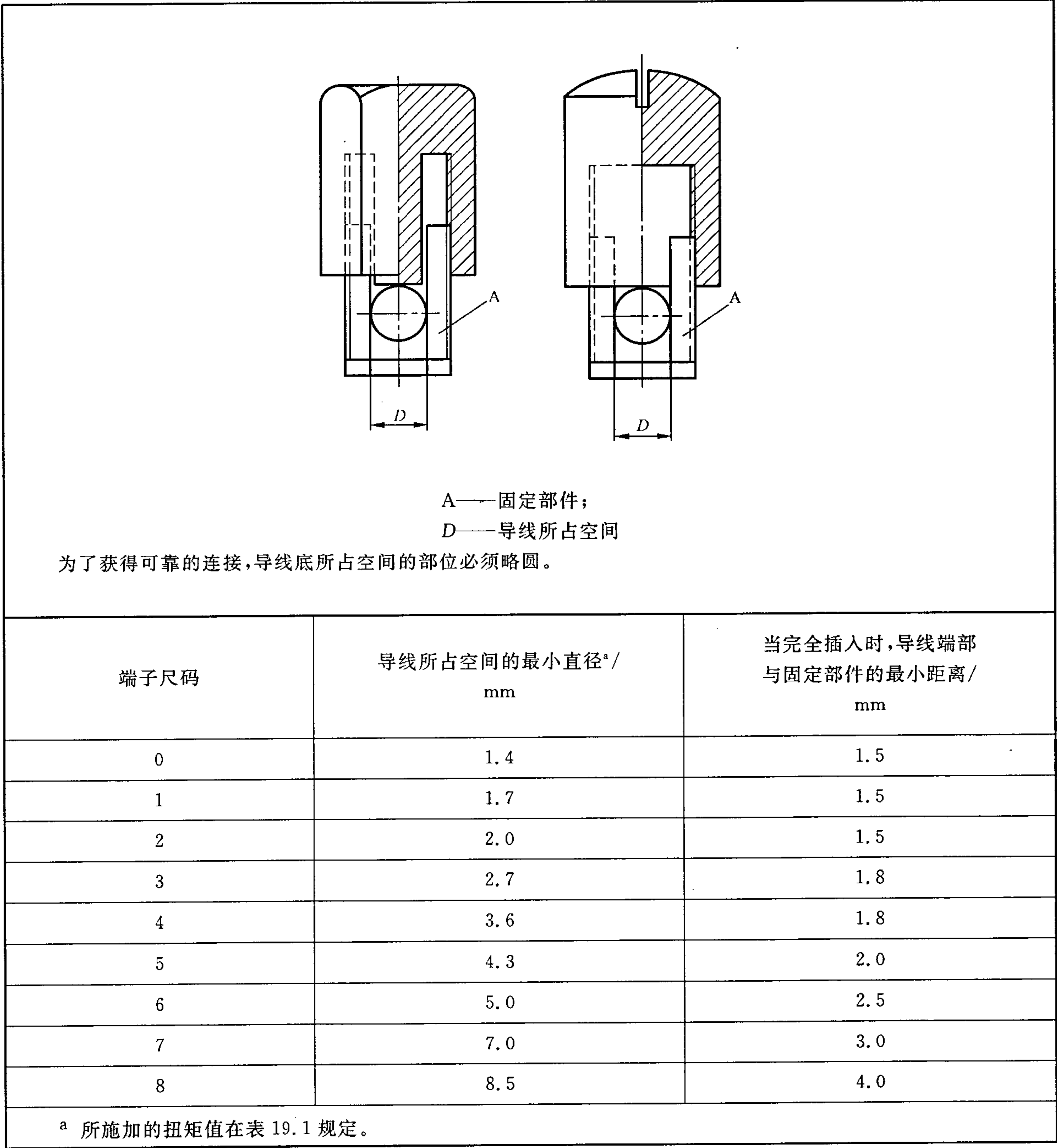
图 12 罩形端子
