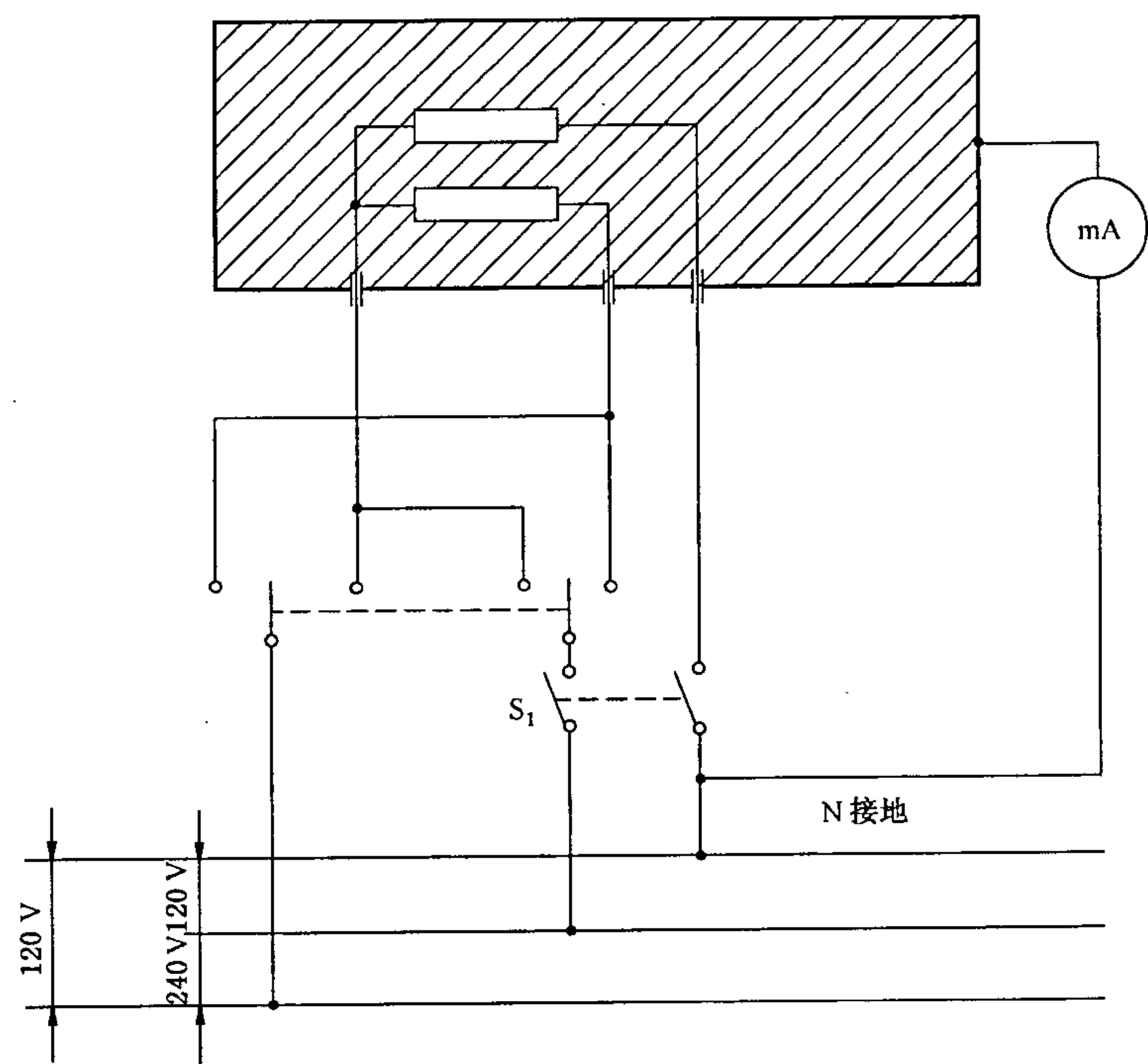
图 30 在工作温度下测量非 II 类控制器在二相连接到三相中线接地电源上时泄漏电流的接线图
