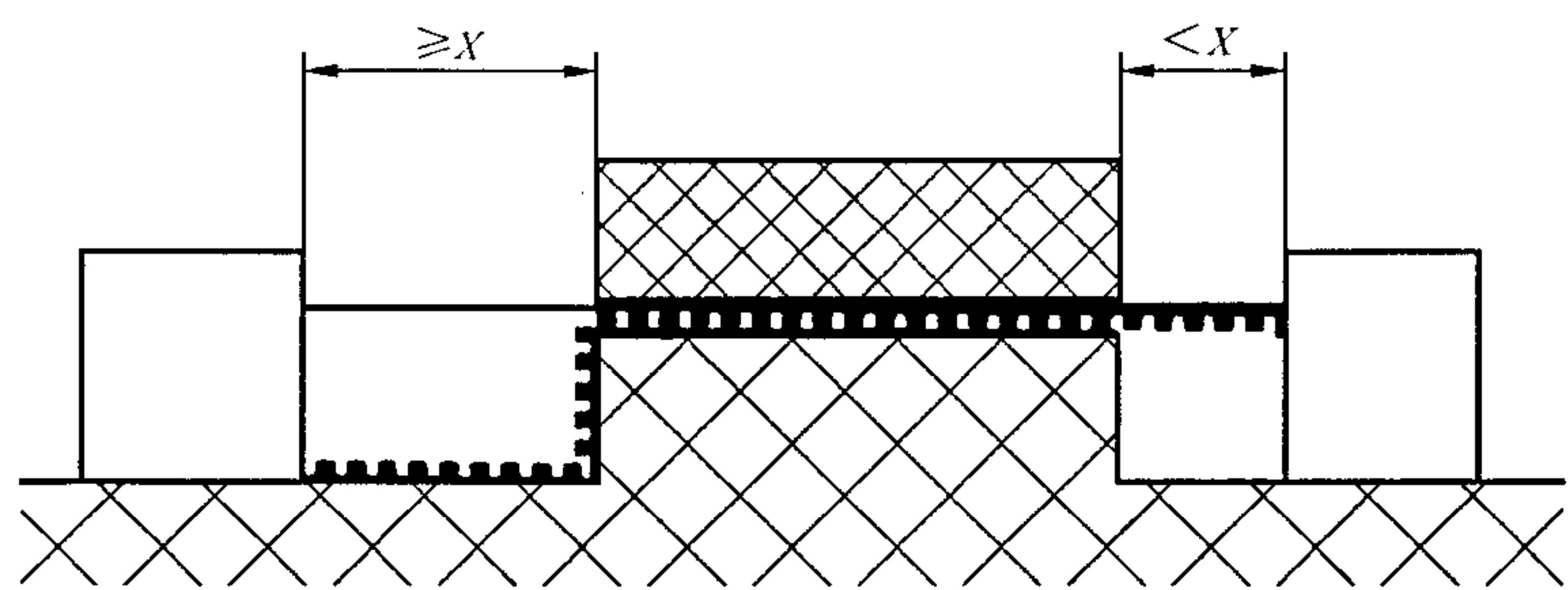
注：所考虑的路径包括一个未粘固的结合处和一个宽度小于 X 的槽及一个宽度等于或大于 X 的槽。 规则：间隙路径和爬电距离路径如图所示。
