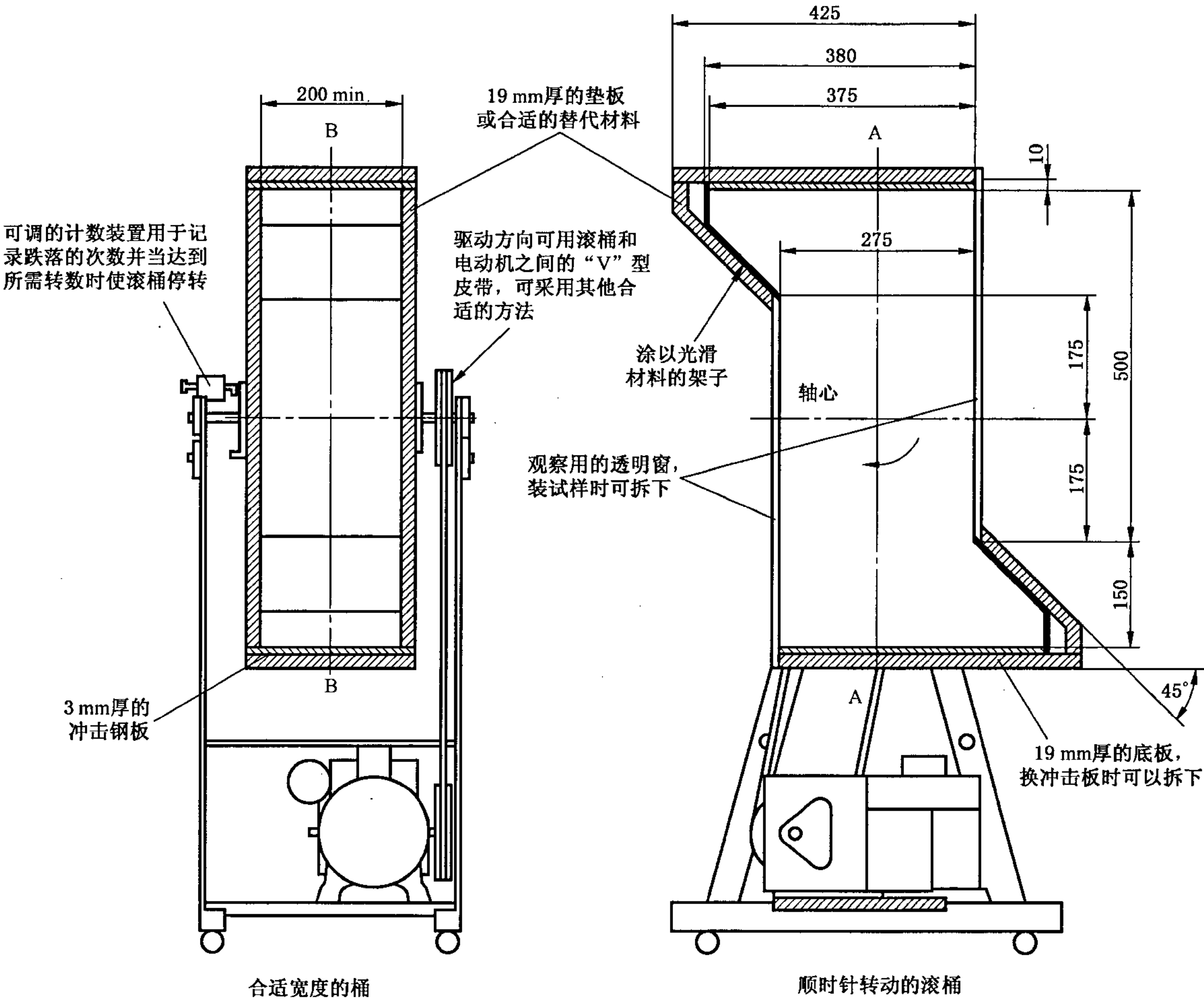
图5 滚桶
