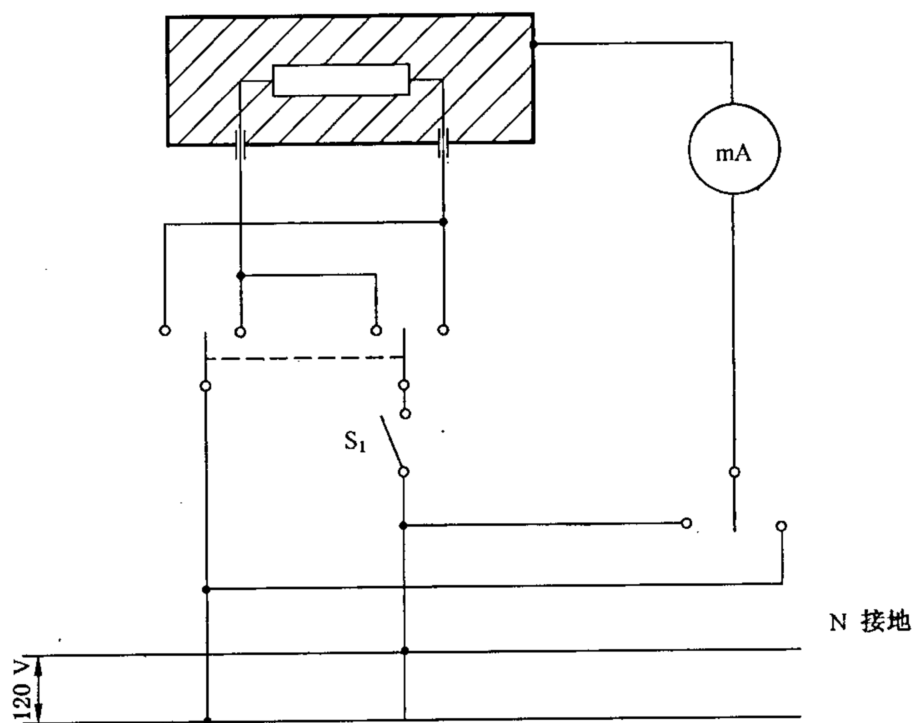
图 26 在工作温度下测量非Ⅱ类控制器在单相连接时泄漏电流的接线图
