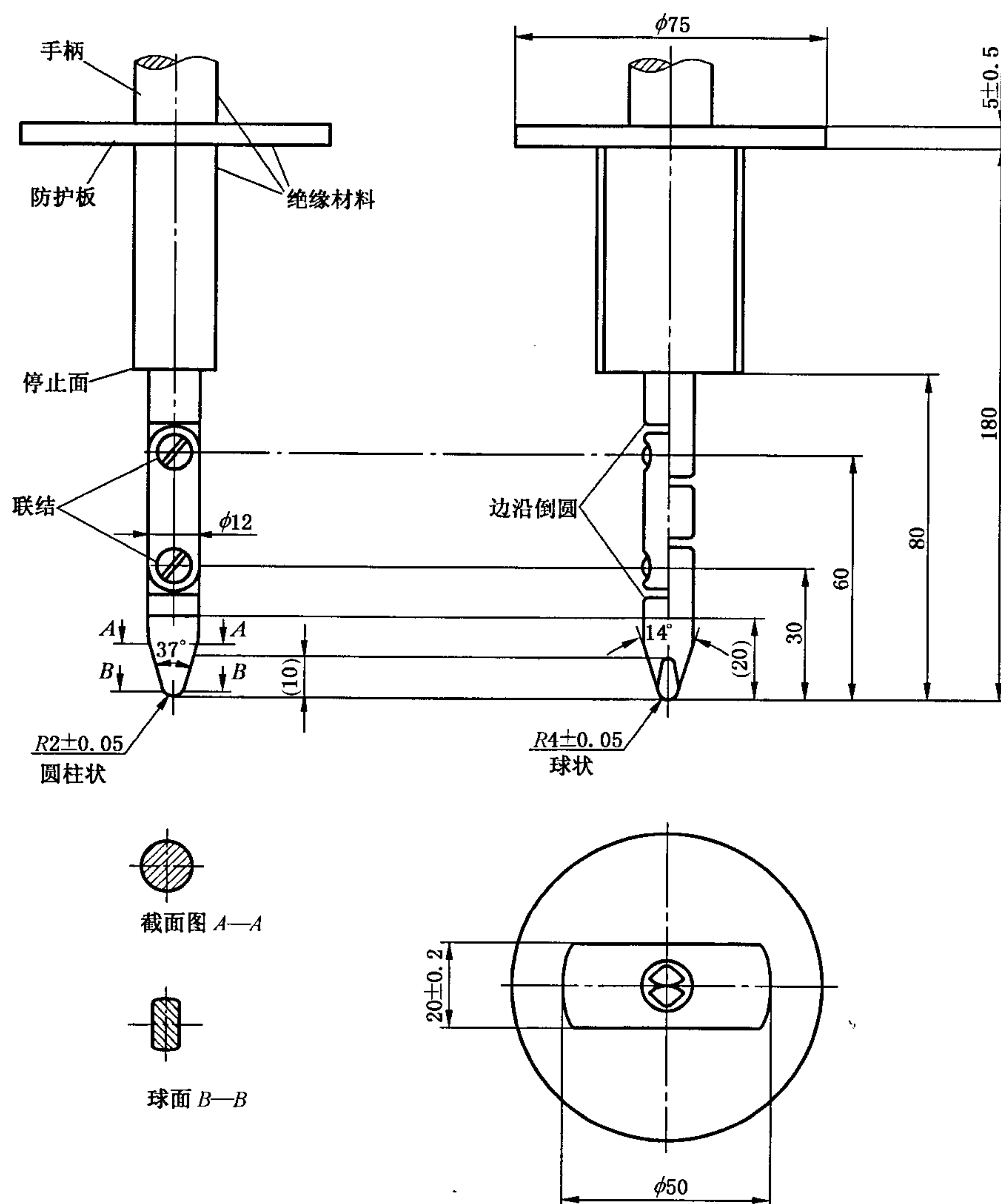
图 1 试验针
