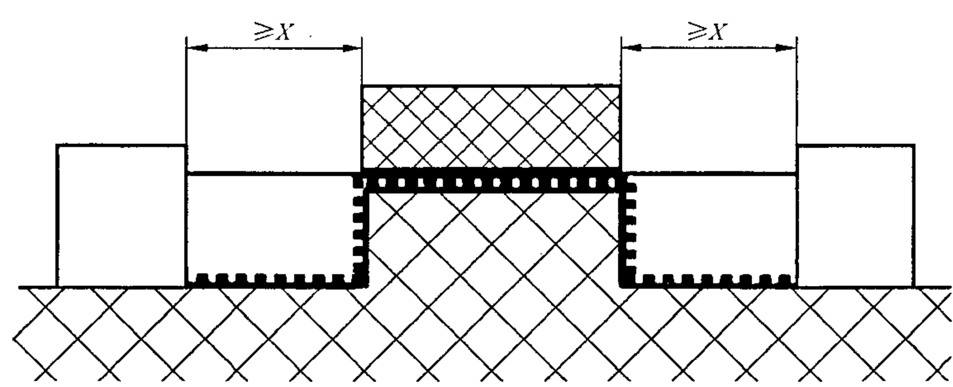
注：所考虑的路径包括一个未粘固的结合处及一边一个宽度大于 X 的槽。 规则：间隙路径是“视线”路径。 爬电距离路径是沿槽的轮廓路径。
