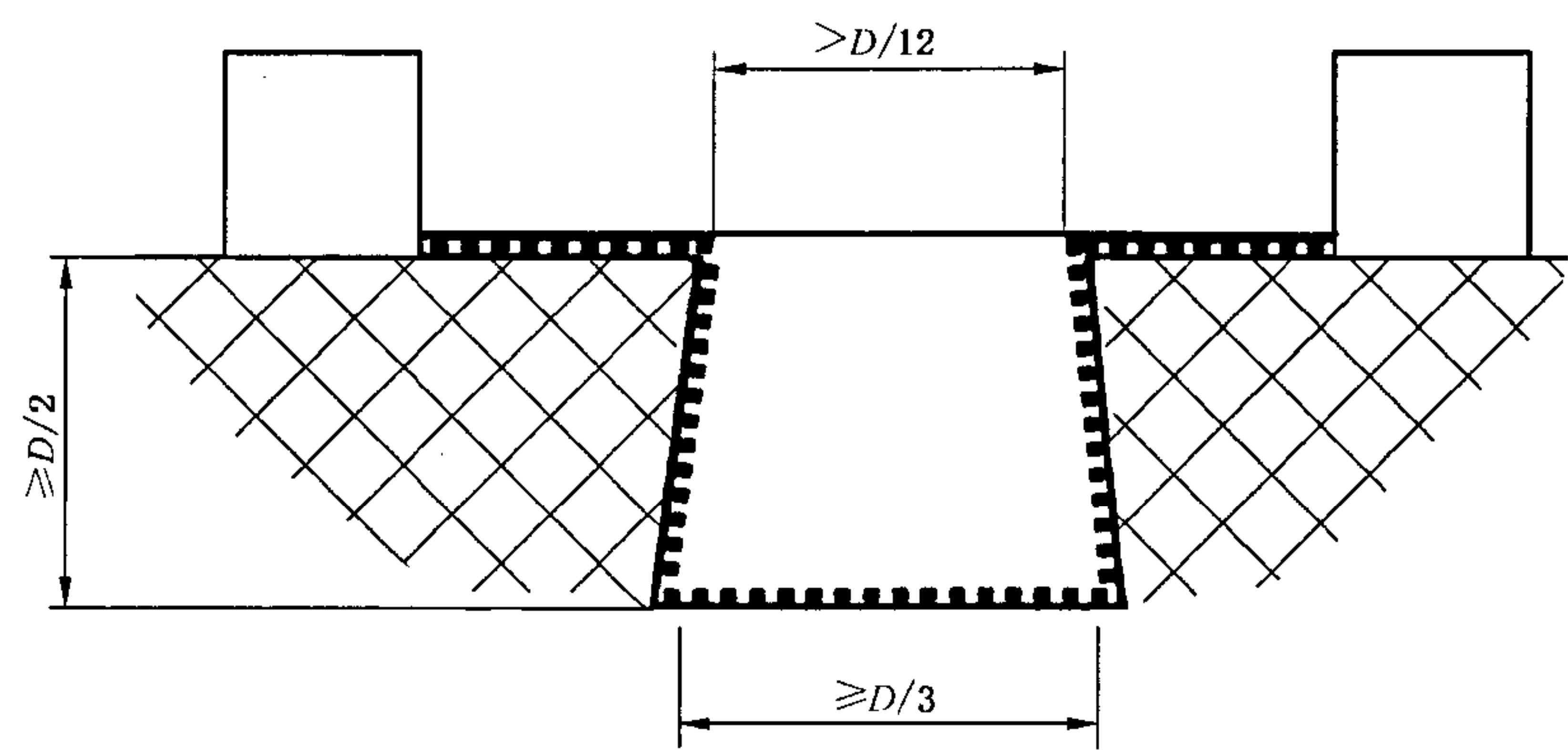
注：所考虑的路径包括两壁发散的槽，其深度等于或大于 D/2 而最窄部分的宽度超过 D/12 ，底部等于或大于 D/3 。 规则：间隙路径是“视线”路径。 爬电距离路径沿槽的轮廓。 如果内角小于 80^\circ ，图 B. 3 的规则也适用于内角。
