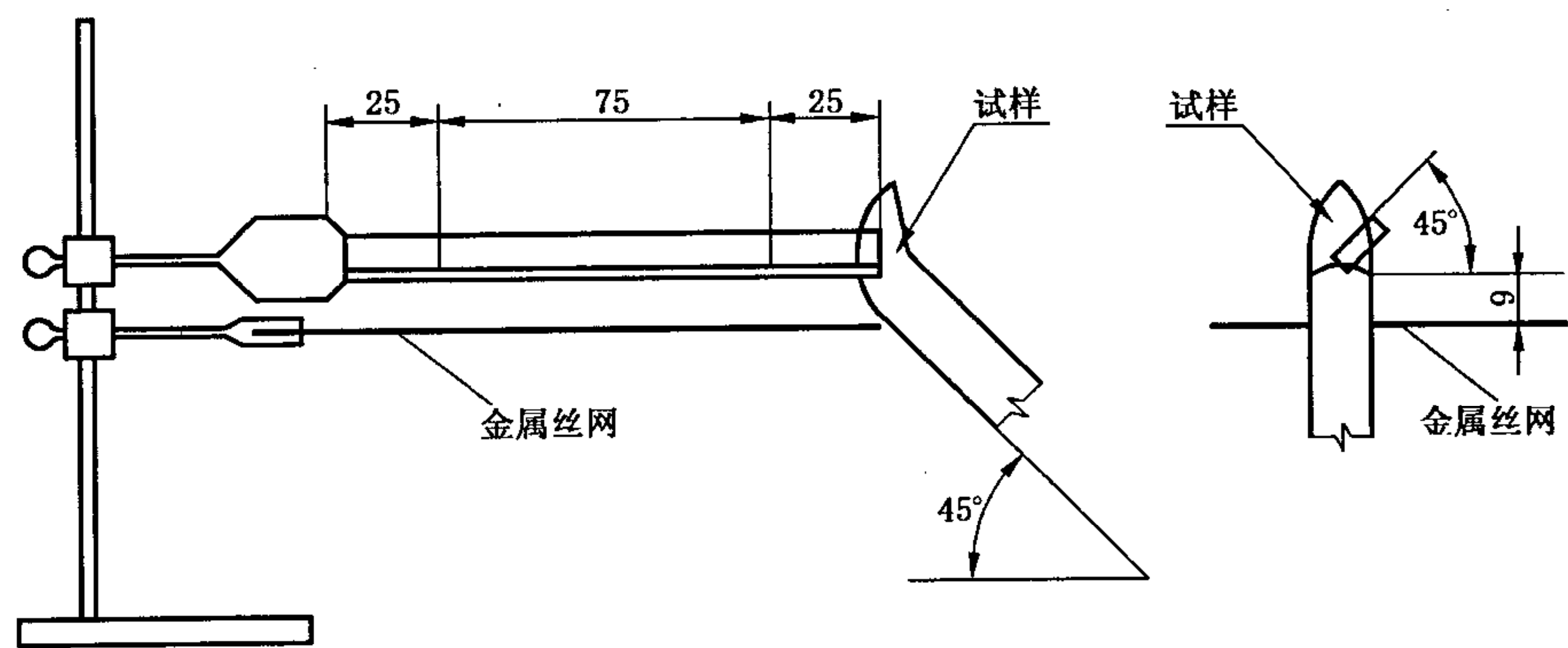
图 7 水平燃烧试验
