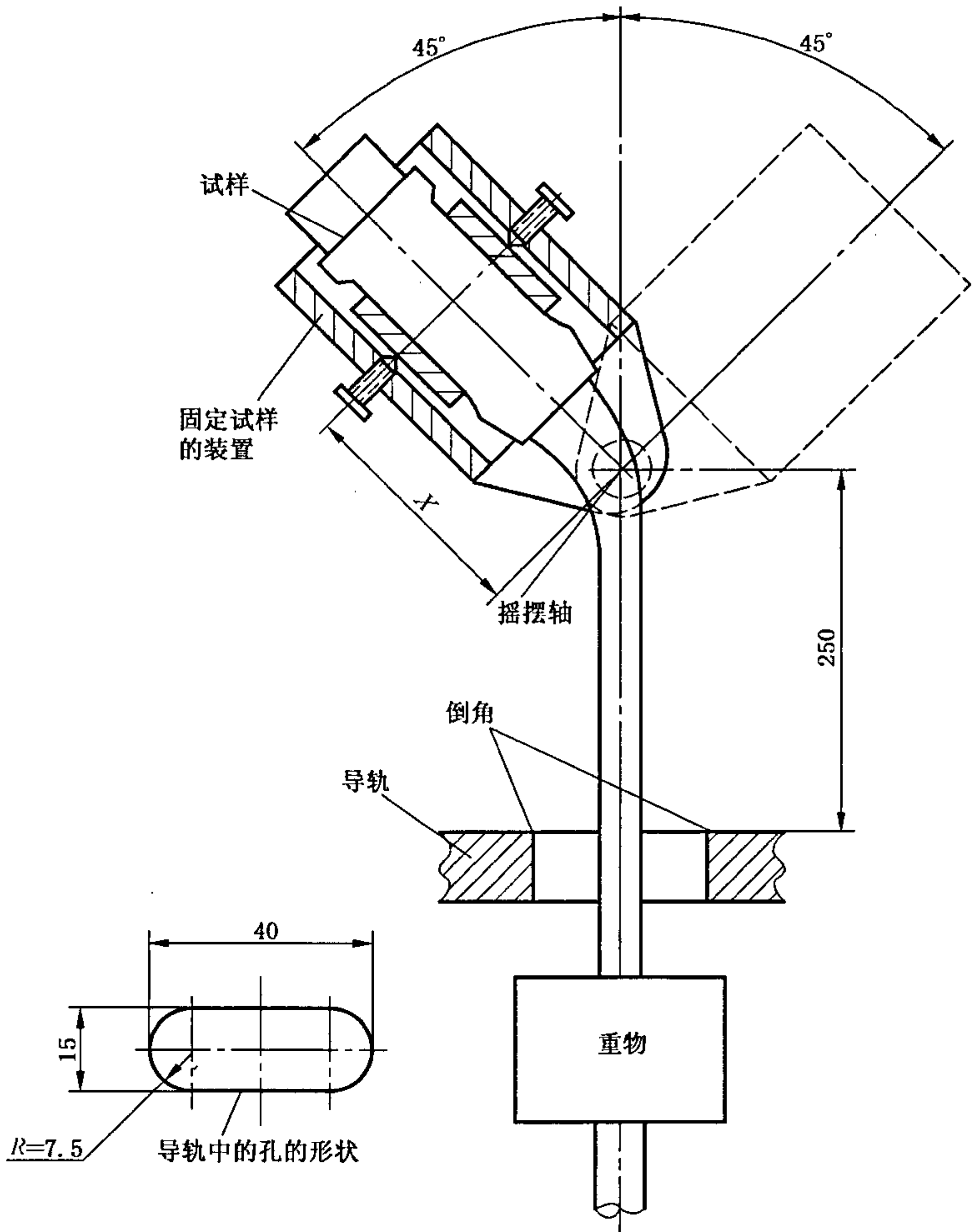
图 9 弯曲试验设备
