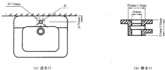
图 C.3 洗面器和净身器
