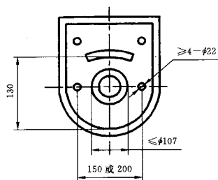
(b) 后排式坐便器
