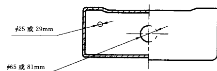
图 C.4 水箱
