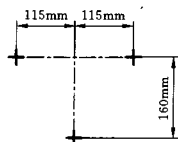
(b) 3孔
