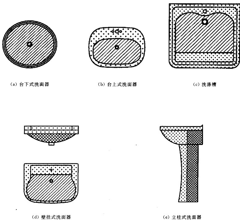
图 B.1 洗面器及洗涤槽表面区域划分示意图
