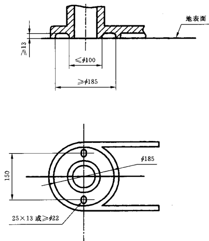
(a) 下排式坐便器
