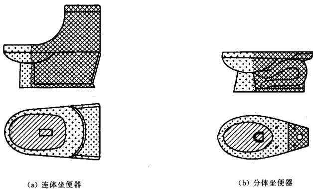
图 B.2 坐便器表面区域划分示意图
