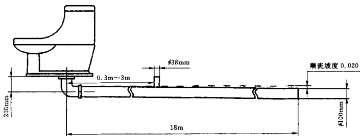
(a) 下排式坐便器
