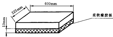
(a) 试验板
