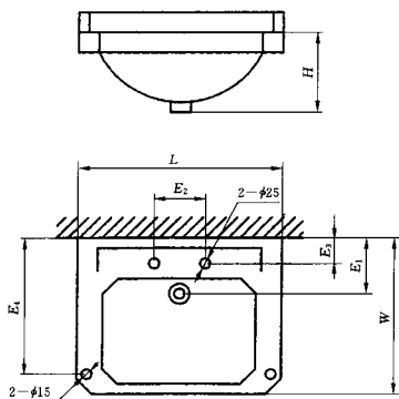
(a) 单孔洗面器
