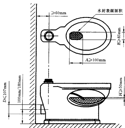
图 C.2 坐便器(二)
