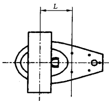
(a) 试验板
